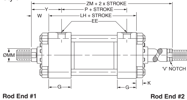
Rod End #1
